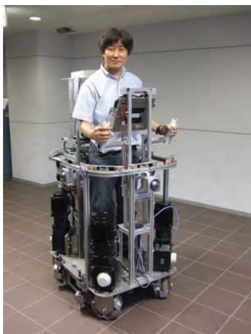
全方位に移動できる個人用知的移動体のプロトタイプ Personal Intelligent Vehicle Capable of Omni-Directional Movement
