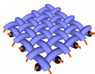
圧力分布を検知できる織物の構造
